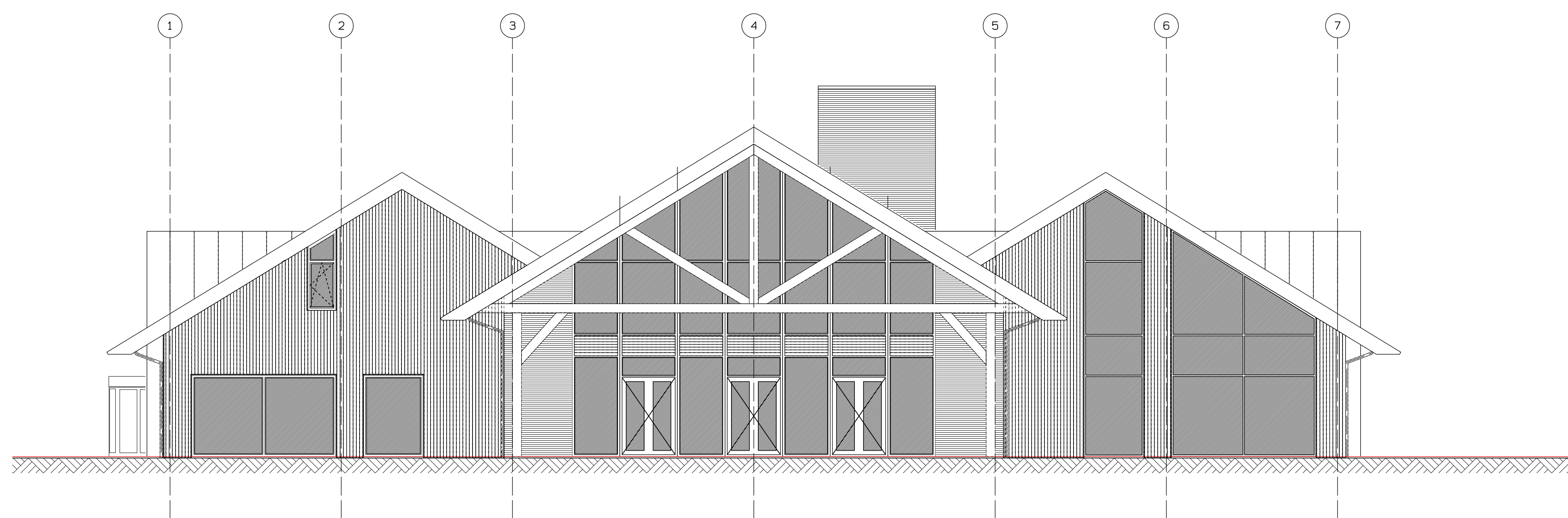
○ GEVELAANZICHT VANAF BREDASEWEG
