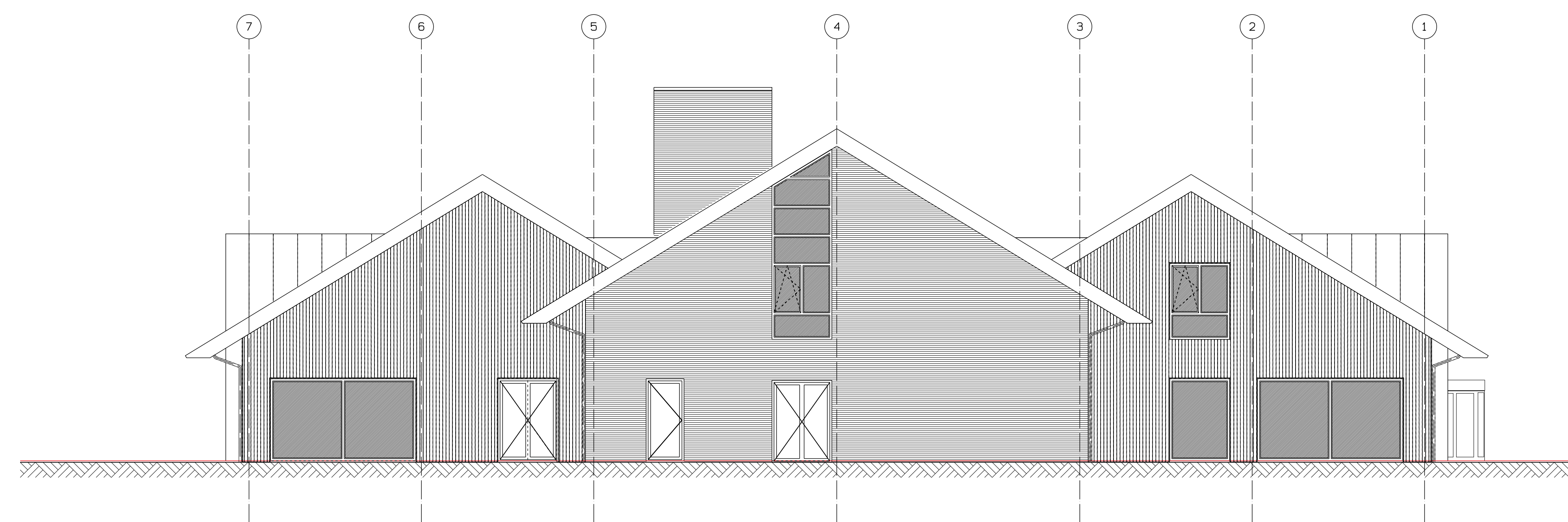
○ GEVEL VANAF VLAGTWEDDESTRAAT
